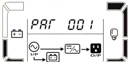
Рисунок 21 – Показания LCD-дисплея при параллельной работе ИБП
