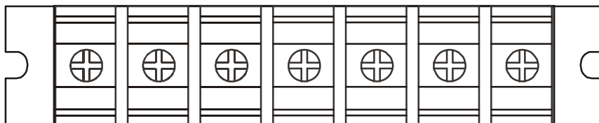
Рисунок 5 – Внешний вид клеммного блока ИБП ATS 10000 3/1 T-X (R)
