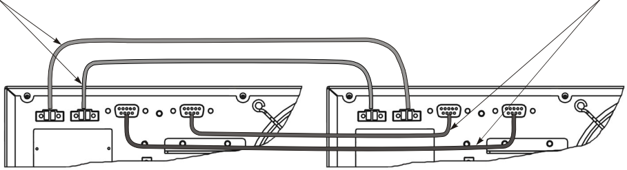
Рисунок 23 – Подключение информационных кабелей к двум ИБП в параллельной системе
