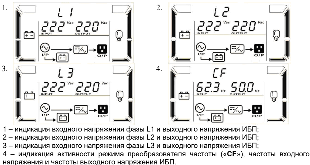
Рисунок 17 – Показания LCD-дисплея ИБП в режиме преобразователя частоты
