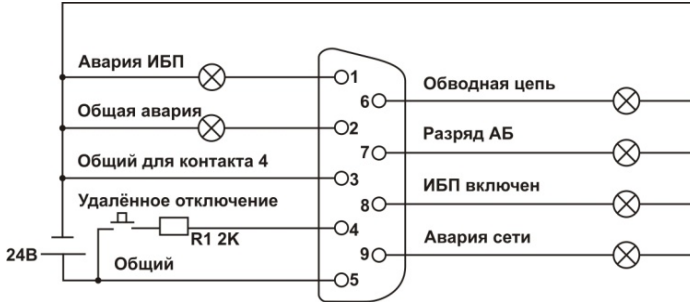
Рисунок 7 – Электрическая схема организации контроля и управления ИБП с электропитанием от источника постоянного тока напряжением +24 В
