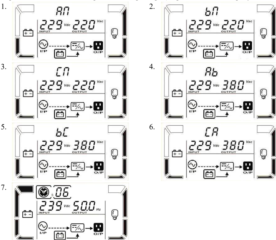
Рисунок 16 – Показания LCD-дисплея ИБП в режиме тестирования батарей На рисунке 16 представлены:
