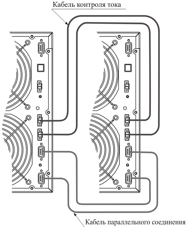
Рисунок 21 – Подключение информационных кабелей к двум ИБП в параллельной системе
