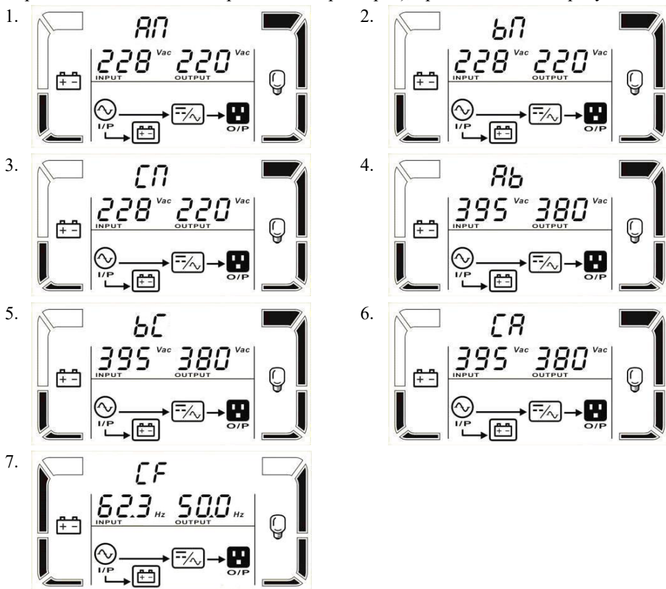
Рисунок 15 – Показания LCD-дисплея ИБП в режиме преобразователя частоты На рисунке 15 представлены:
