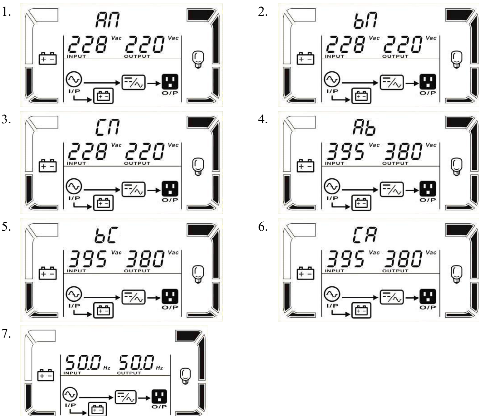
Рисунок 13 – Показания LCD-дисплея ИБП в дежурном режиме
