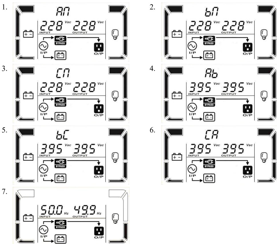
Рисунок 12 – Показания LCD-дисплея в режиме работы ИБП по встроенной обводной цепи
