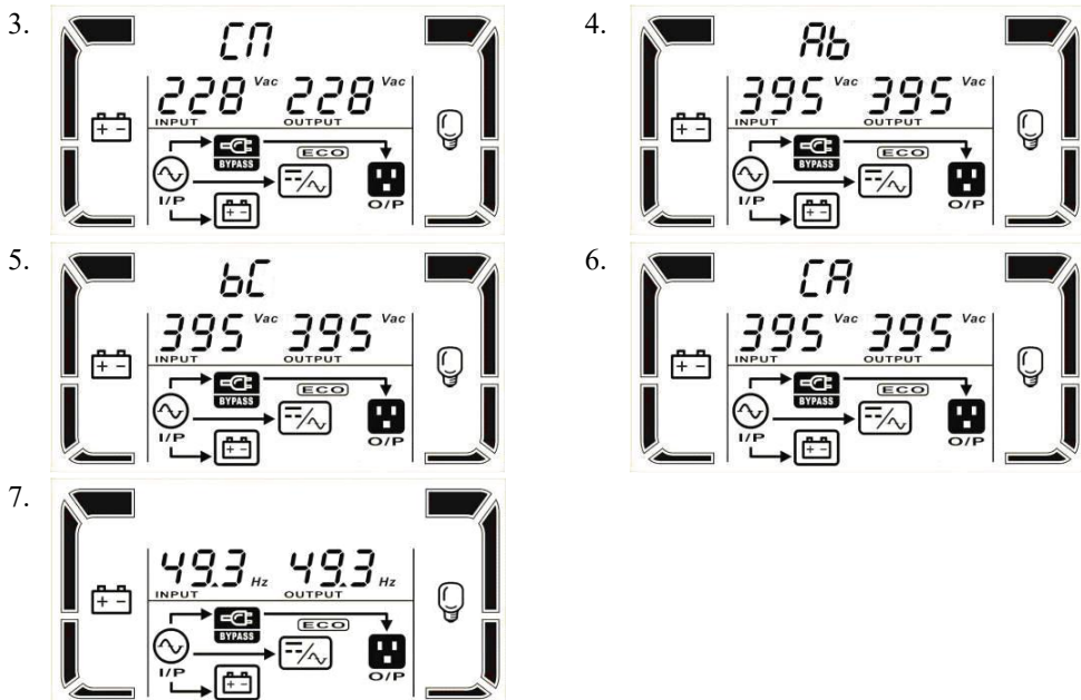
Рисунок 17 – Показания LCD-дисплея ИБП в режиме экономии энергии
