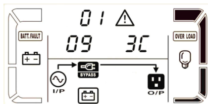
Рисунок 18 – Показания LCD-дисплея ИБП с кодами предупреждающих сообщений
