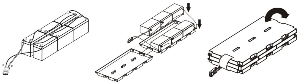
Рисунок 21 – Последовательность установки аккумуляторов в контейнер ИБПАТС 3000 R-VE
