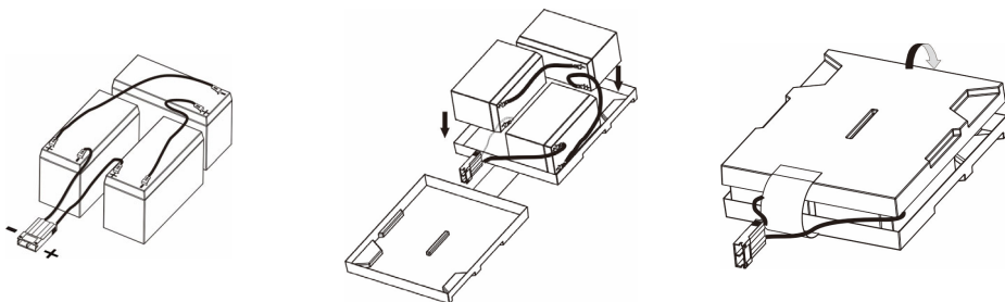
Рисунок 19 – Последовательность установки аккумуляторов в контейнер ИБПАТС 1000 R-VE, ATS 1500 R-VE
