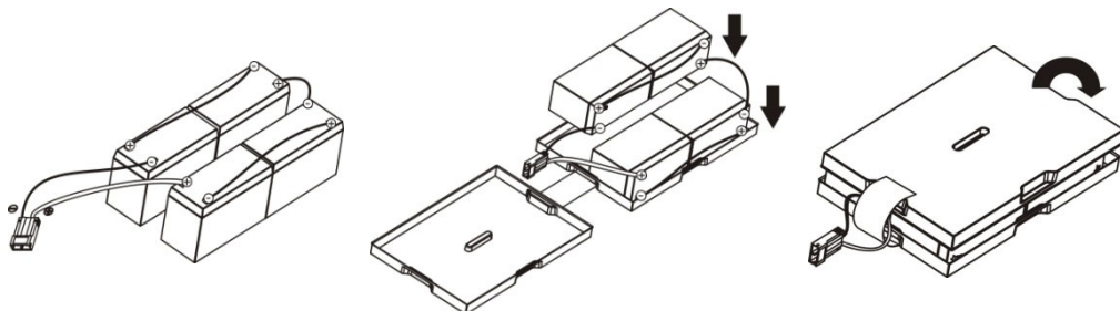
Рисунок 20 – Последовательность установки аккумуляторов в контейнер ИБПАТС 2000 R-VE
