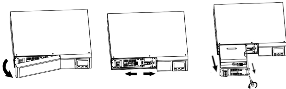
Рисунок 18 – Последовательность извлечения контейнера с батареями из корпуса ИБП
