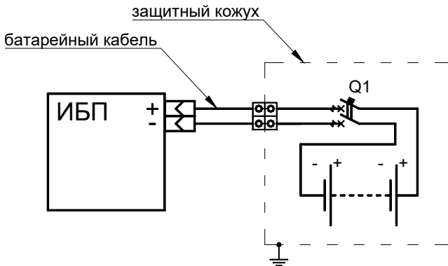
Рисунок 11 – Схема электрическая подключения аккумуляторной батареи к ИБП
