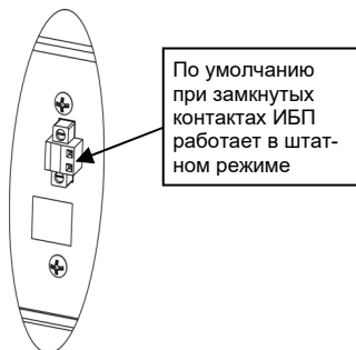
Рисунок 13 – Внешний вид порта дистанционного аварийного отключения (ЕРО), расположенного на задней панели ИБП
