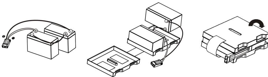
Рисунок 19 – Последовательность установки батарей в контейнер ИБП ATS 1000 R-VX, ATS 1000 R-VX (S)
