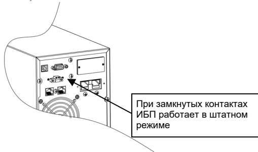
Рисунок 6 – Внешний вид порта дистанционного аварийного отключения (EPO), расположенного на задней панели ИБП
