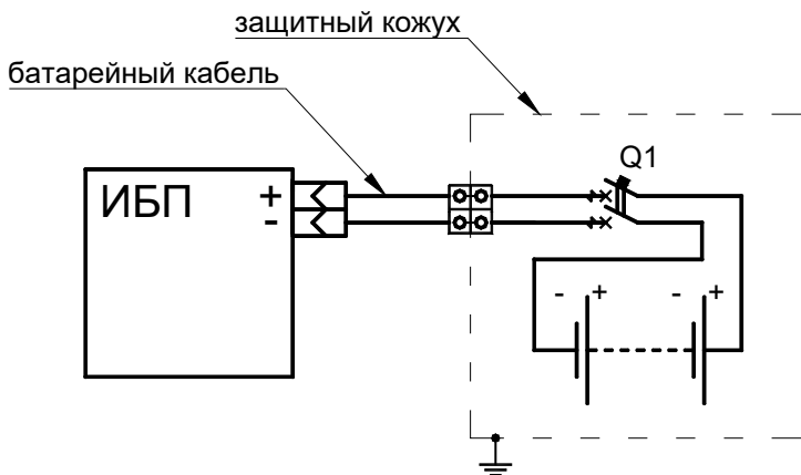
Рисунок 11 – Схема электрическая подключения аккумуляторной батареи к ИБП
