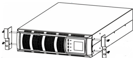
Рисунок 5 – Порядок установки ИБП в стандартный шкаф или стойку для телекоммуникационного оборудования шириной 19 дюймов
