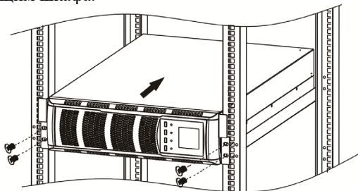
Рисунок 5 – Порядок установки ИБП в стандартный шкаф или стойку для телекоммуникационного оборудования шириной 19 дюймов
