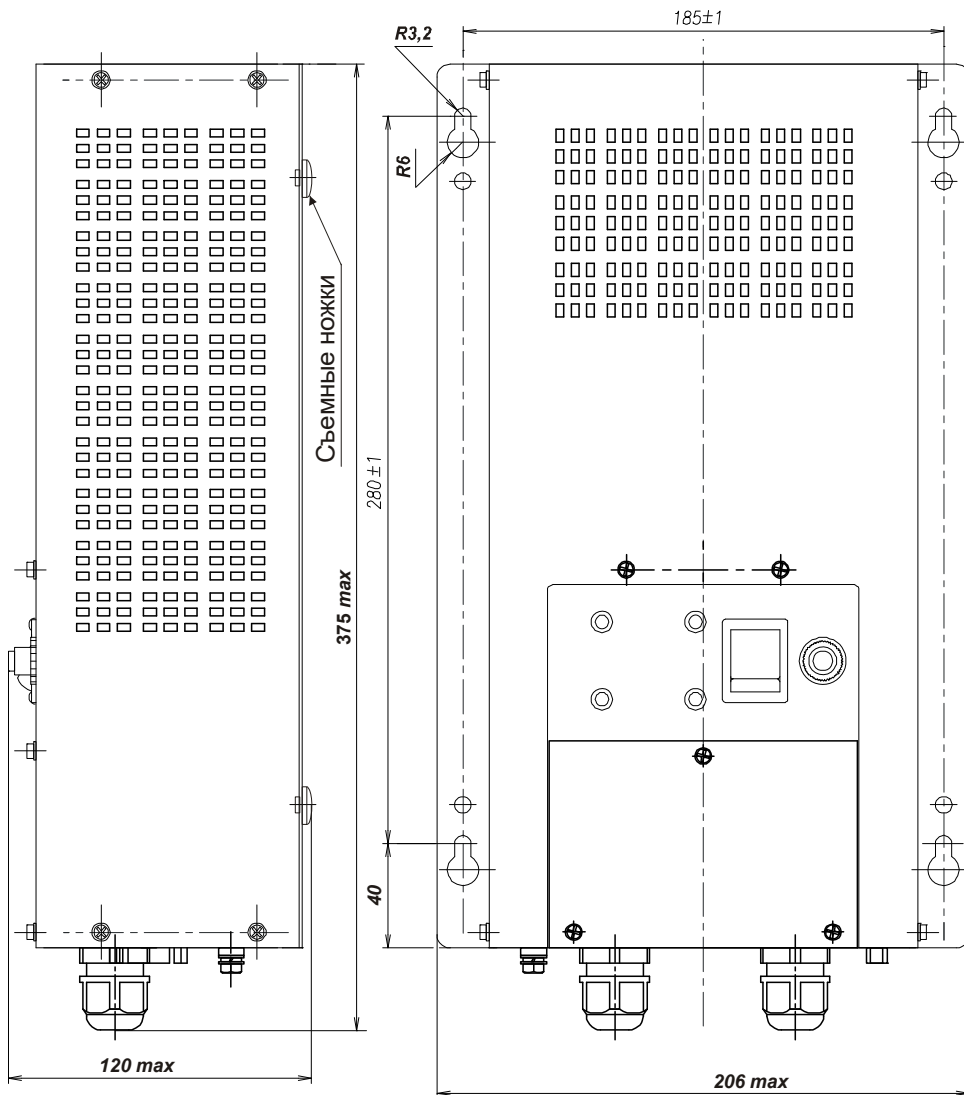
Рисунок А.1 – Габаритные и установочные размеры стабилизатора
