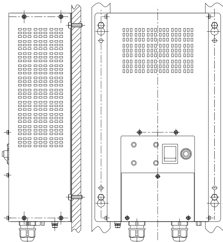
Рисунок Б.1 – Монтаж стабилизатора на вертикальную плоскость (стену) или другие вертикальные несущие конструкции (удалить съемные ножки перед монтажом)
