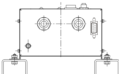
Рисунок Б.2 – Монтаж стабилизатора на горизонтальную плоскость или другие горизонтальные несущие конструкции (удалить съемные ножки перед монтажом)
