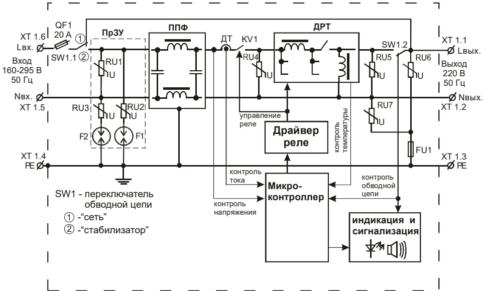
Рисунок 2 – Упрощённая структурная схема стабилизатора
